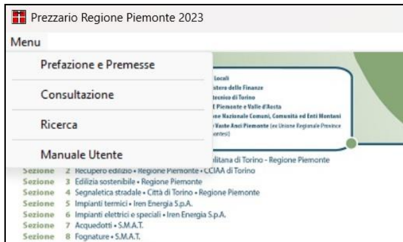
Figura 2: Menu funzionalità
